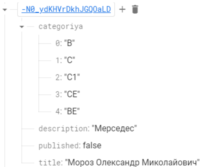
Рис. 2.4. Структура таблиці drivers.
