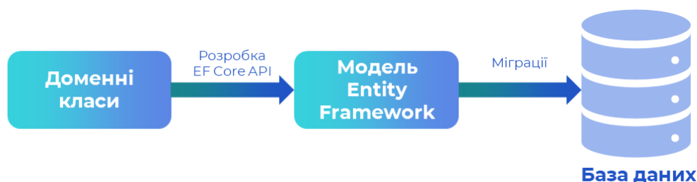
Рис. 5.3. Міграції в Entity Framework Core
