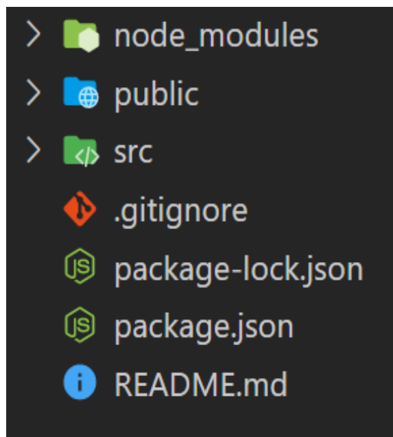
Рис. 6.4. Структура Front-End
