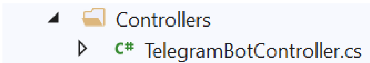
Рис. 6.9. Контролер телеграм-бота
