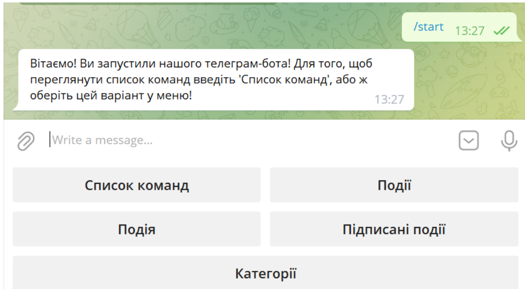
Рис. 8.9. Команда «/start»
