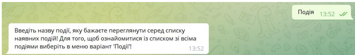
Рис. 8.17. Команда «Подія»
