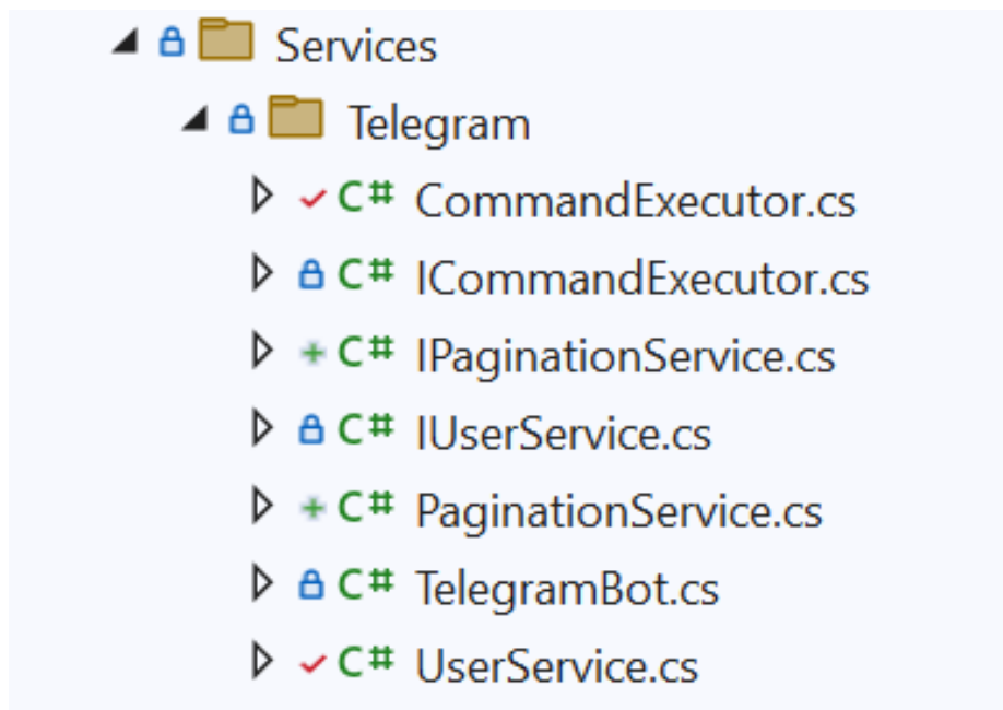
Рис. 6.10. Сервіси
