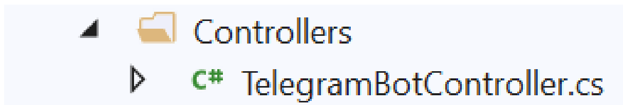
Рис. 6.9. Контролер телеграм-бота
