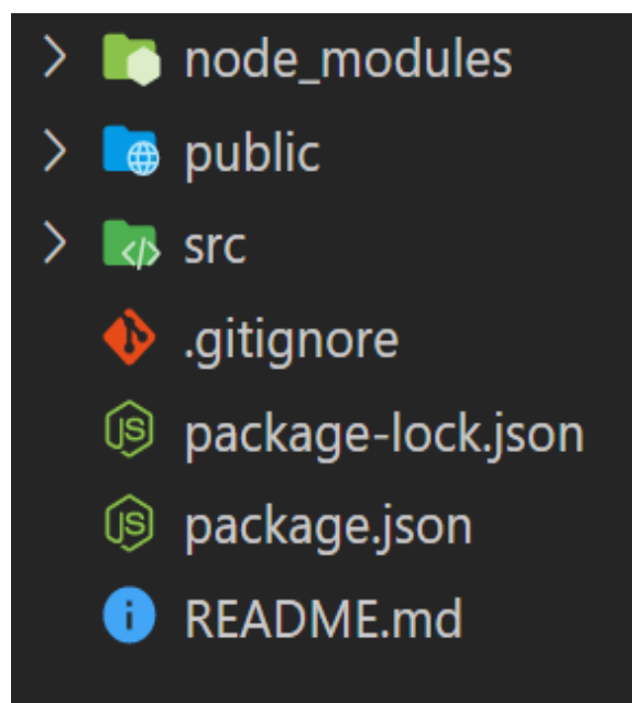
Рис. 6.4. Структура Front-End
